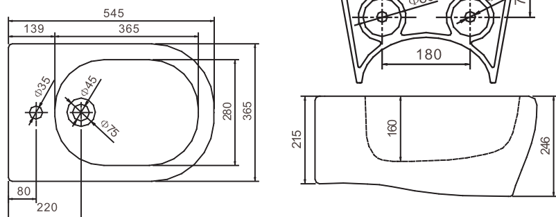
CB-5005 Unit:mm
